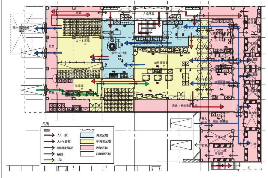
図2 ゾーニングと空気の動線
