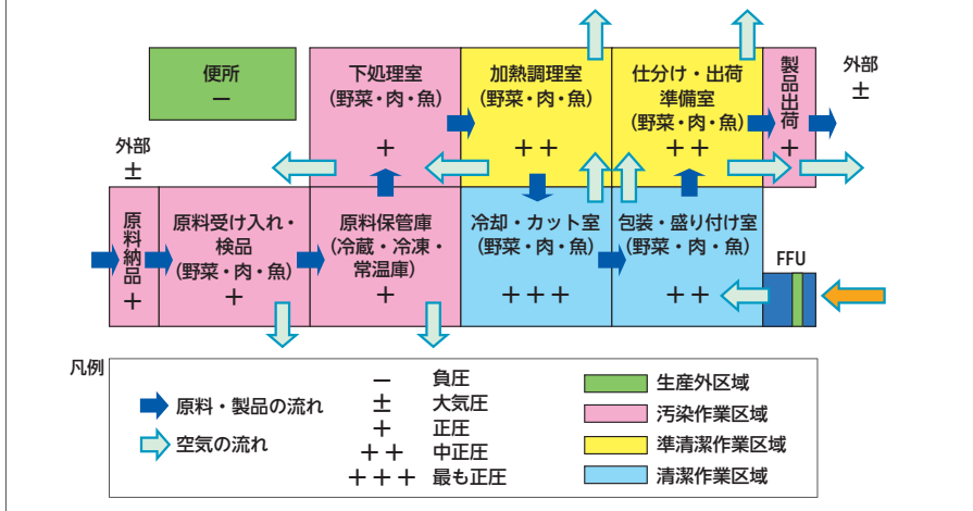
図3 ゾーニングと気流・室圧(陽圧管理)
