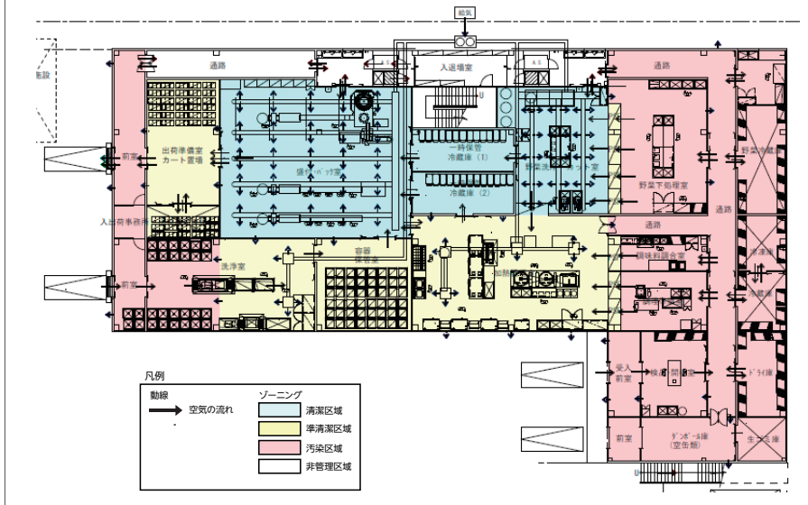
図3 ゾーニングと気流・室圧(陽圧管理)
